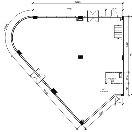
MẶT BẰNG TẦNG 1
