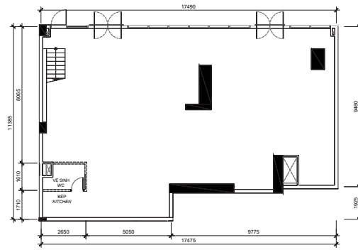
MẶT BẰNG TẦNG 1
