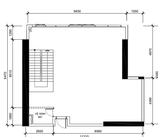
MẶT BẰNG TẦNG 2
