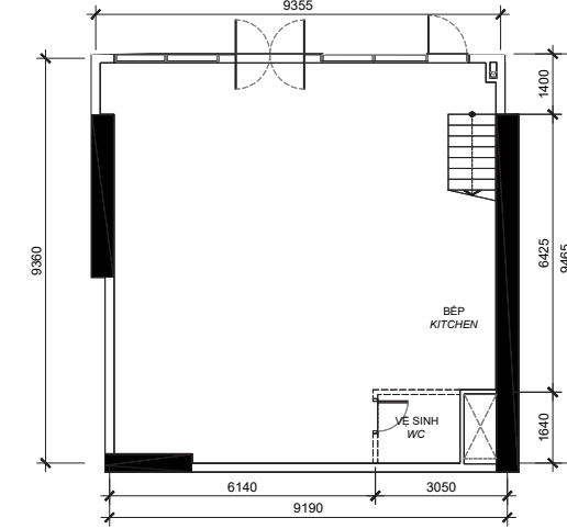
MẶT BẰNG TẦNG 1
