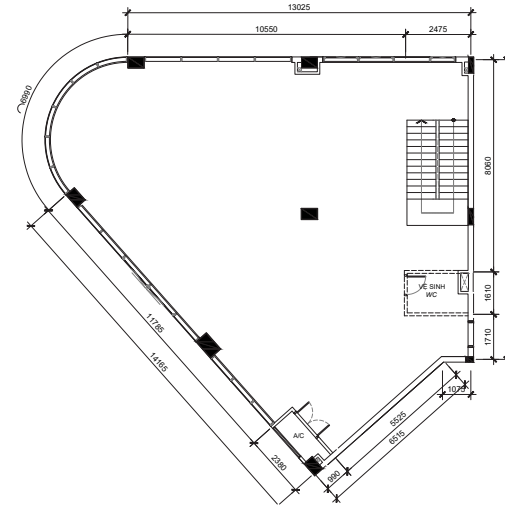
MẶT BẰNG TẦNG 2
